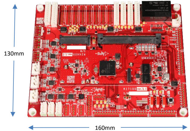
※写真はNPE製コントロールカードK24409 _TMS320F28379DZWT(TI)を接続した状態です。
