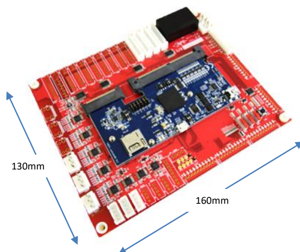
※写真はTI製コントロールカード (TMDSCNCD28379D)を接続した状態です。
